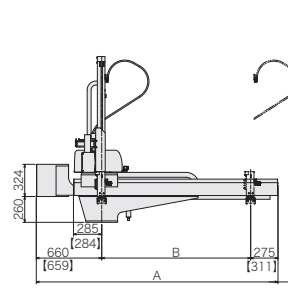
■操作側取出規格
