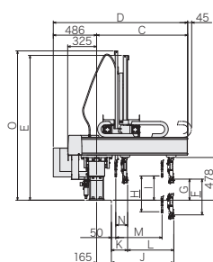
■反操作側取出規格
